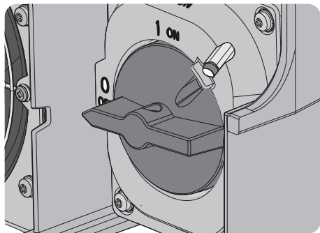
Imagen 3.2. Interruptor-seccionador fotovoltaico
