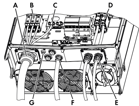
Abbildung 5.2 Überblick über Wechselrichter mit Drehmomentvorgaben
