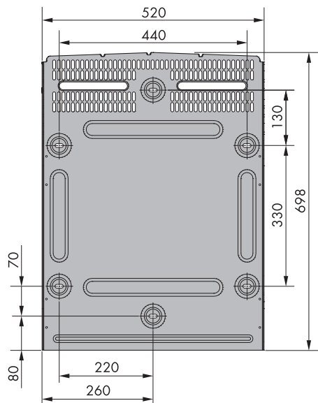
Figura 2.9 Dimensioni del supporto da parete in mm
