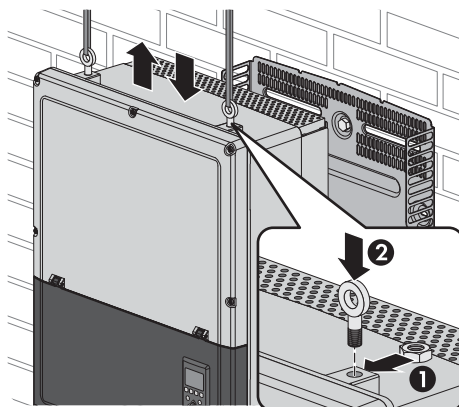
Figure 2.11 : Fixation des boulons en U et levage de l'onduleur
