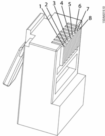
Abbildung 5.4 Pinbelegung des RJ45-Steckers für Ethernet
