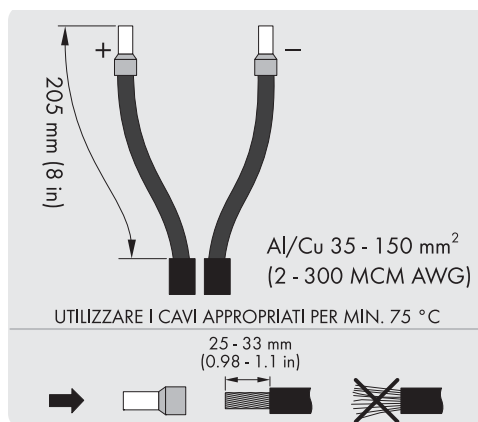
Figura 2.24 Adesivo FV
