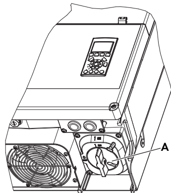
Abbildung 1: PV-Lasttrennschalter
