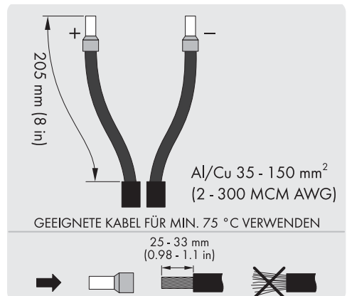
Abbildung 2.24 DC Aufkleber
