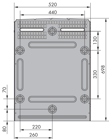
Figure 2.9 : Dimensions du support mural en mm
