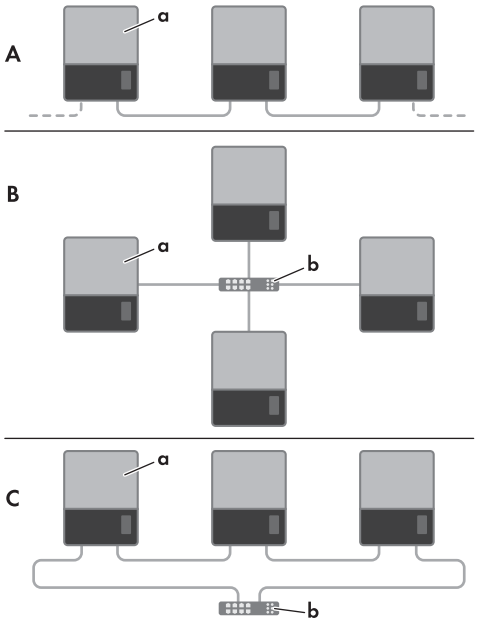
Imagen 5.5. Topología de red
