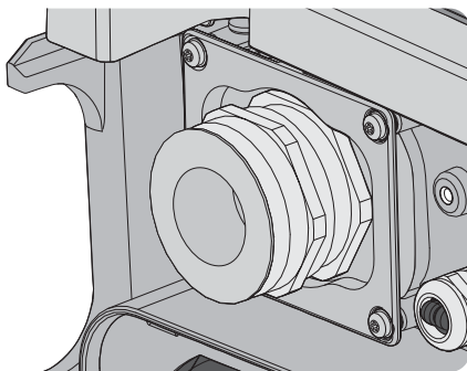
Figure 2.18 : Presse-étoupe AC
