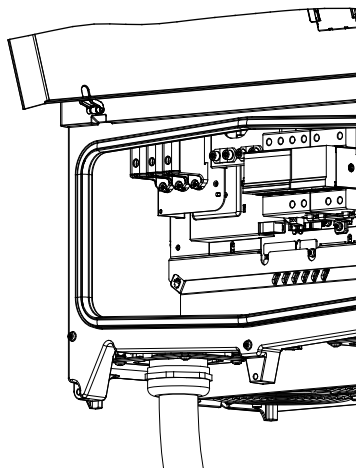
Imagen 2.14. Área de instalación
