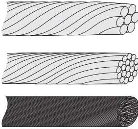
Abbildung 2.16 Kabel mit verschiedenen Leitern (von oben nach unten): mehrdrähtig, feindrähtig und feindrähtig
