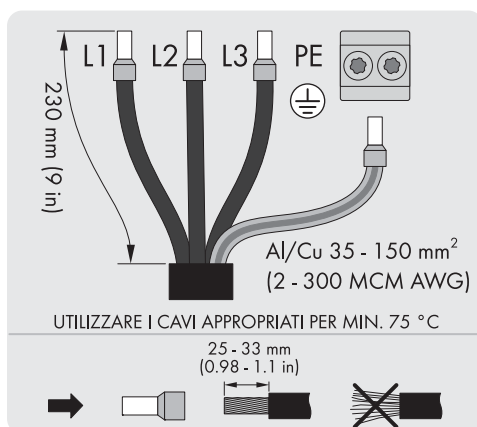
Figura 2.15 Spelatura del cavo CA
