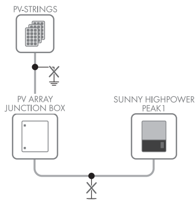
Figure 2.21 : NE PAS relier le raccordement photovoltaïque à la terre
