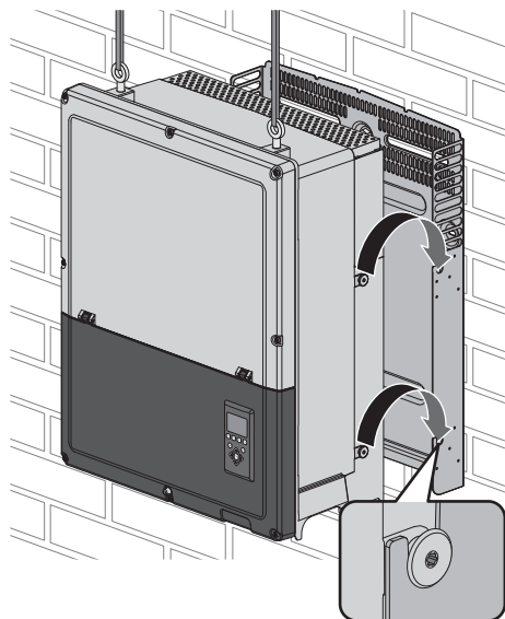
Figura 2.12 Cuelgue el inversor de red aislado en el soporte mural.
