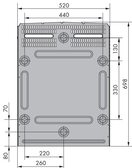
Imagen 2.9. dimensiones del soporte mural en mm
