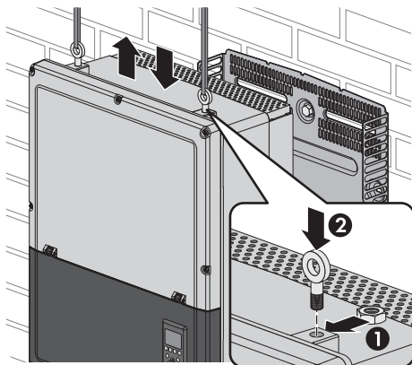
Imagen 2.11. Fije las argollas de elevación y levante el inversor
