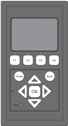
Figura 3.1 Panoramica dei pulsanti del display e relative funzioni
