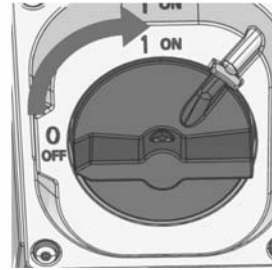
Abbildung 3.2 PV-Lasttrennschalter
