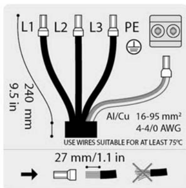
Figura 2.17 Spelatura del cavo CA
