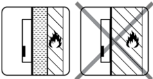
Abbildung 2.5 Auf nicht entflammbarer Oberfläche montieren
