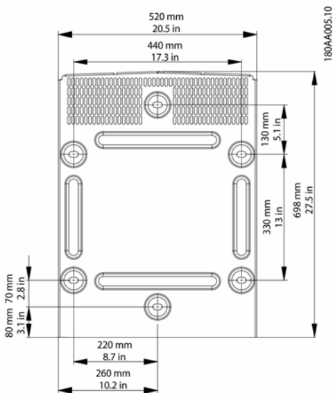
Figura 2.9 Supporto da parete
